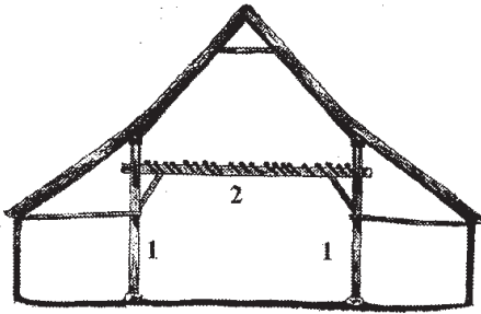
Gebint hallehuis. Kenmerkend is het ankergebint 1 stijl, 2 ankerbalk
